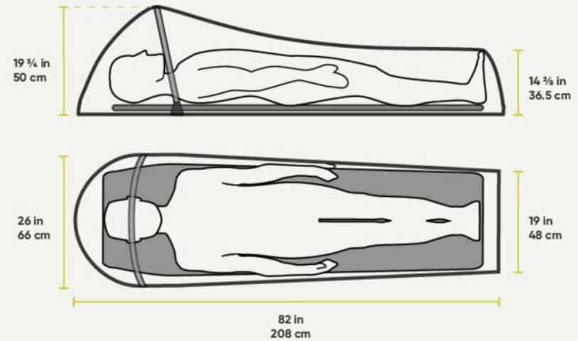
Helium Bivy
