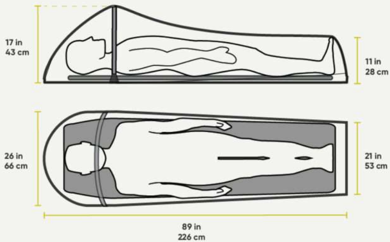
Bug Bivy
